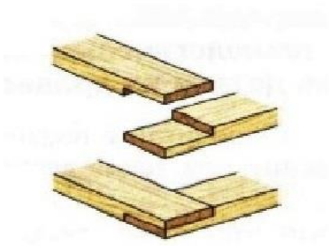
Рисунок №1. Соединение брусков вполдерева (вкладку).
