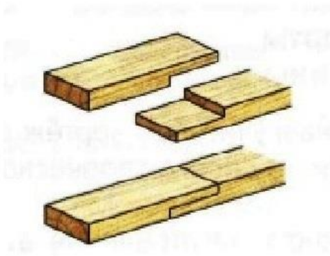
Рисунок №1. Соединение брусков вполдерева (внакладку).
